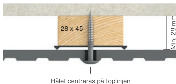
Fig. 2. Swisspearl Patina Inline monterad på träläkt.
