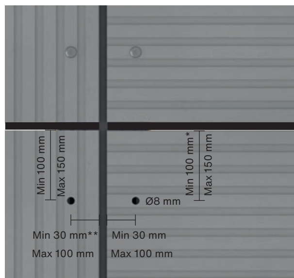
Fig. 3. Swisspearl Patina Inline kant- och hörnavstånd OBS! Minsta avstånd eller närmaste följande toplineje
