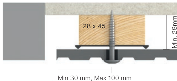
Fig. 4. Swisspearl Patina Inline kantavstånd vid formatkapning
