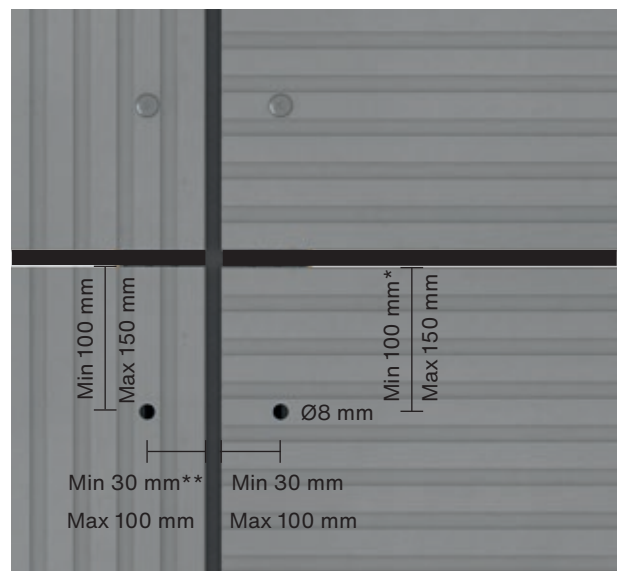
Fig. 3. Swisspearl Patina Inline kant- och hörnavstånd OBS! Minsta avstånd eller närmaste följande topplinje
