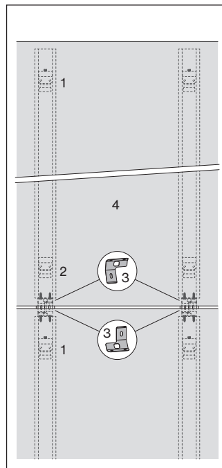
Fassaden-Abschluss oben
