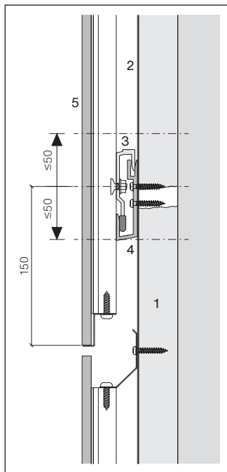
Beispiel Holz-UK
