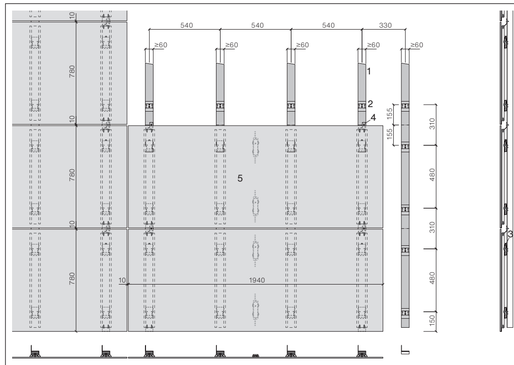
Einteilung Sunskin Facade Flat, Typ XL horizontal, 1940×780 mm
