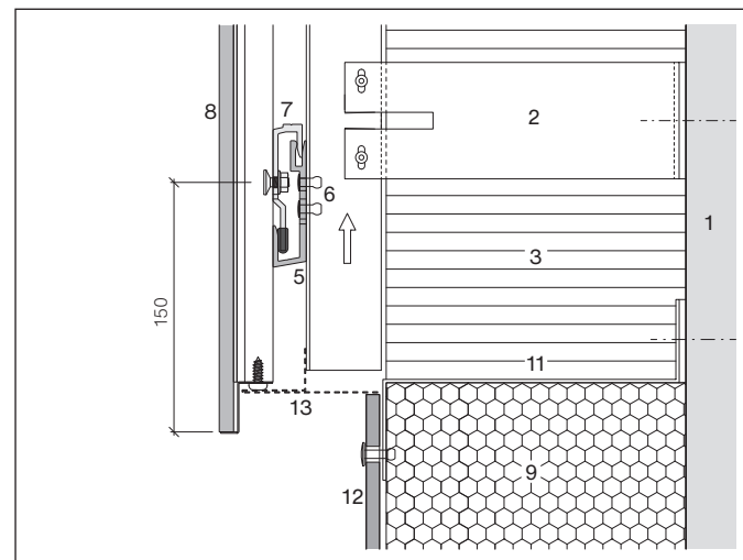
Lösungsvariante mit bauseits abgekanteten Lüftungsprofil
