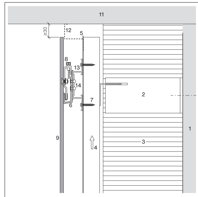
Anschluss Dachuntersicht
