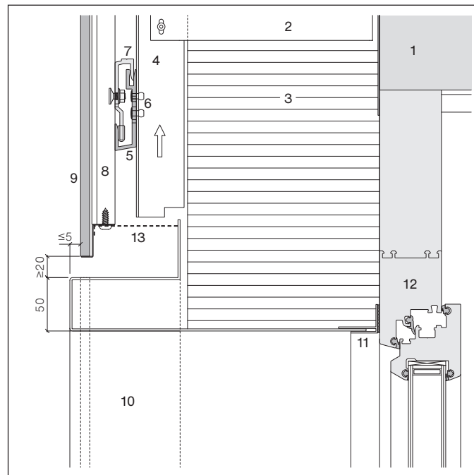
Fenstersturz
