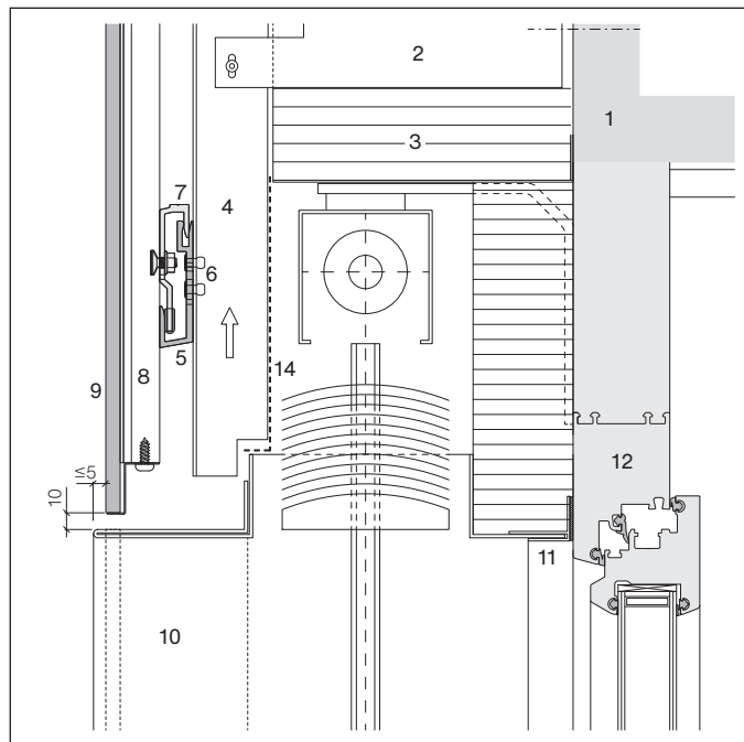
Fenstersturz mit Storenkasten
