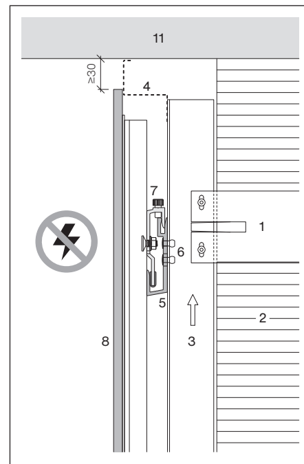
Anschluss Dachuntersicht, Modul inaktiv
