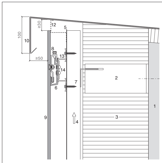
Dachrandabschluss
