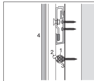
vorderseitige Befestigung
