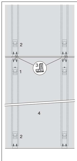
Fassadenfuss
