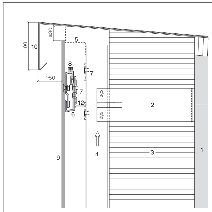
Dachrandabschluss
