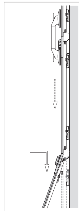
Neue Modul einhängen, befestigen und obere Platte zurücksetzen. Bei Gerüstankern gleiches Vorgehen.
