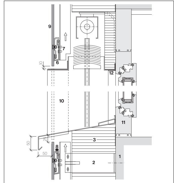
Fensterzarge, Vertikalschnitt
