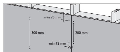
Pagrindiniai atstumai tarp tvirtinimo taškų
