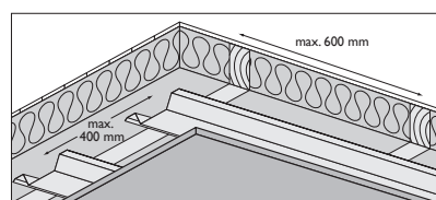
Lubų konstrukcija
