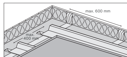
Lubų konstrukcija
