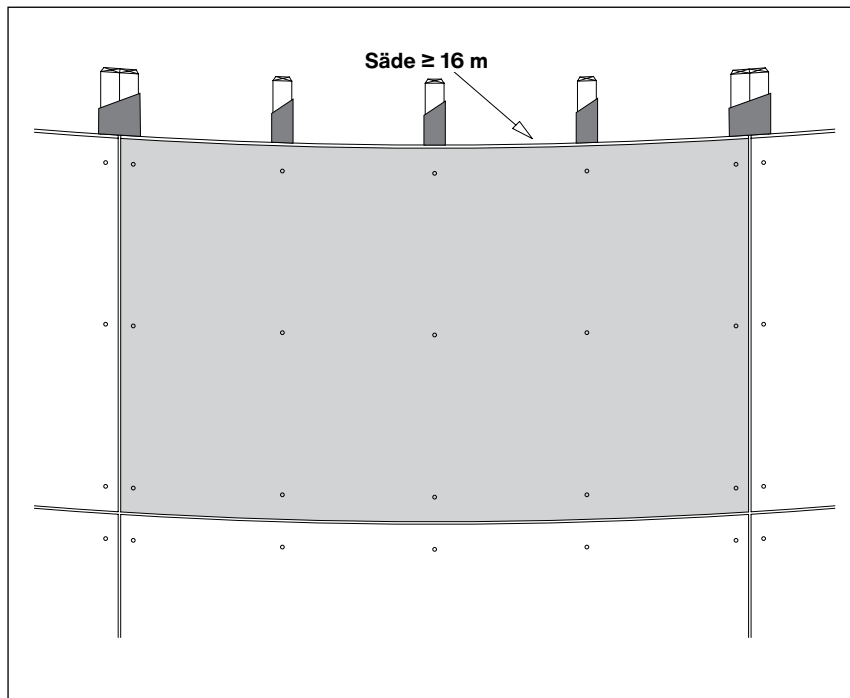
Swisspearl Largo 8 mm, vaakalevytyt
