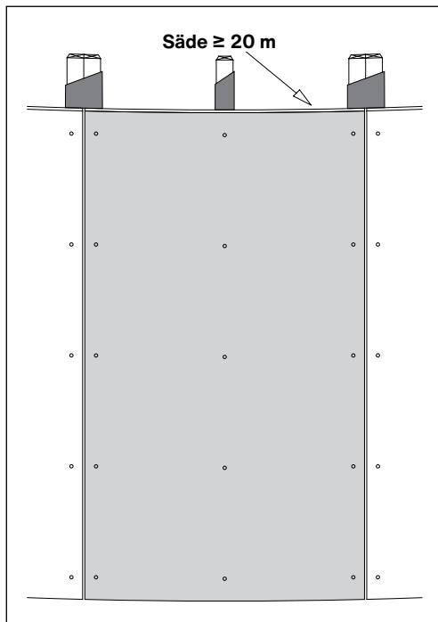
Swisspearl Largo 8 mm, pystylevytyt
