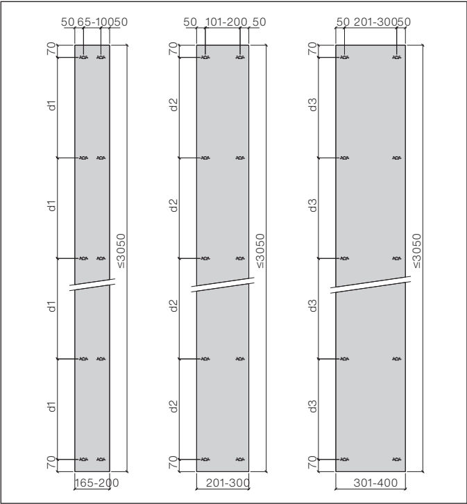
Sigma 8 Pro stroken verticaal aangebracht
