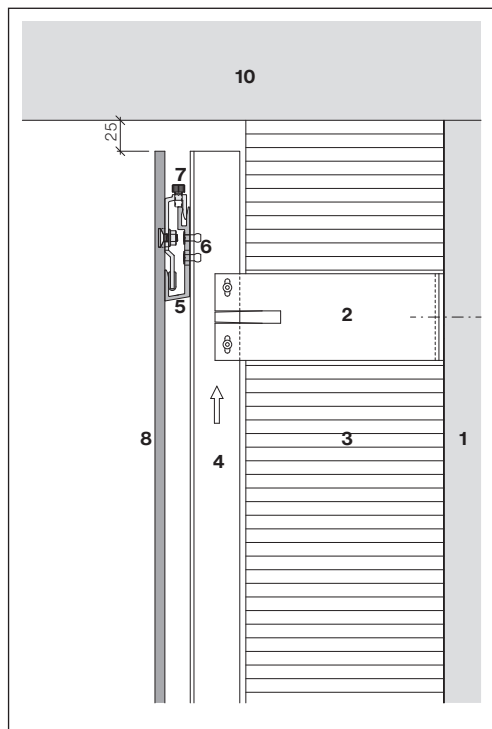
Aansluiting bij het dakoverstek
