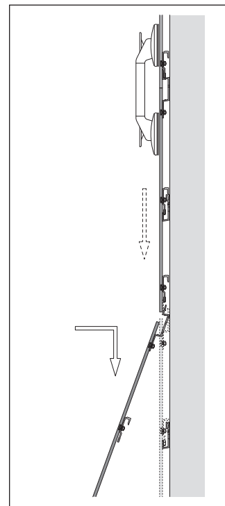
Bevestig een nieuw paneel, zet het bovenpaneel vast en zet het terug. Voor steigerankers geldt dezelfde procedure.
