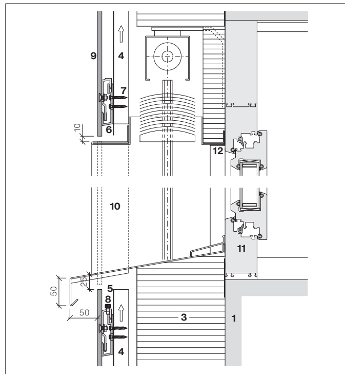
Raamkozijn, verticaal gedeelte
