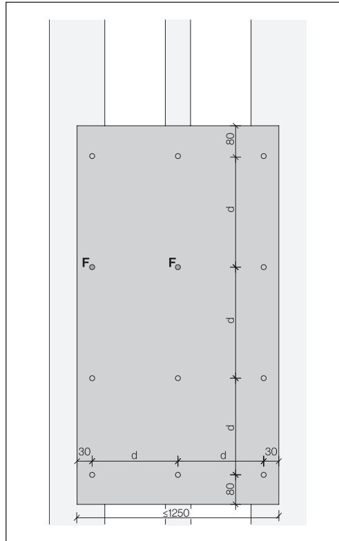
Panneau vertical Swisspearl Largo (portrait)
