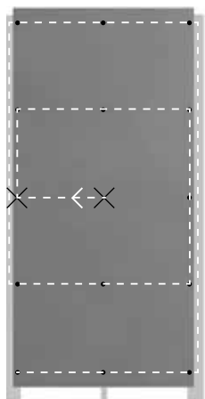
Illustratie van de correcte montageprocedure voor blindklinknagels. 1 en 2 zijn vaste punten
