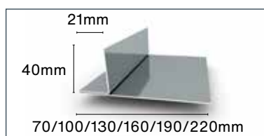
4. Alu verticaal raamprofiel
