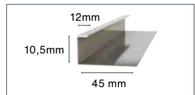
10. Alu eindprofiel Lengte 3055 mm
