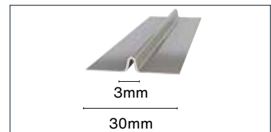
7. Alu voegprofiel Lengte 3055 mm
