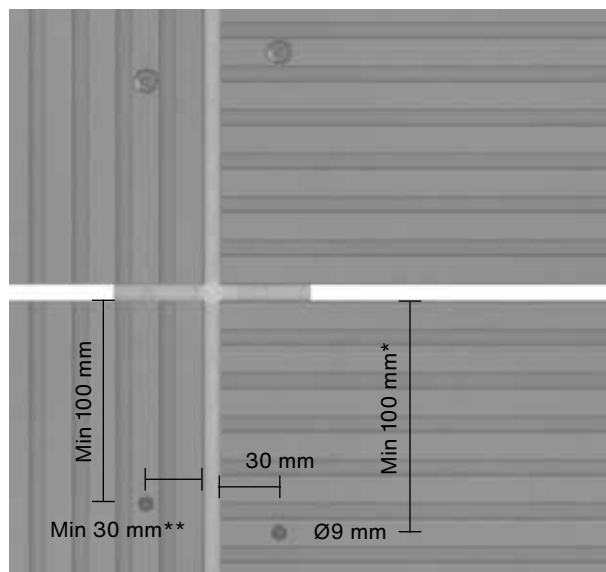
Fig. 3. Swisspearl Patina Inline randafstanden.
