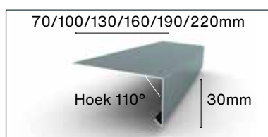
6. Alu raamdorpelprofiel
