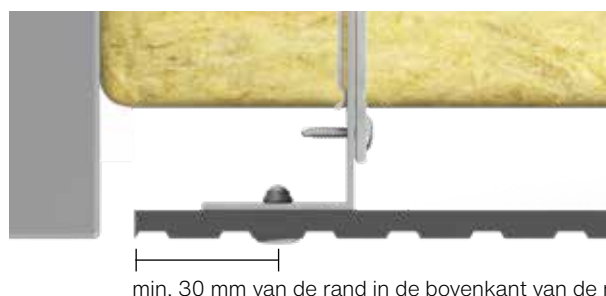
Fig. 4. Swisspearl Patina Inline plaatsing van op maat gezaagde panelen.
