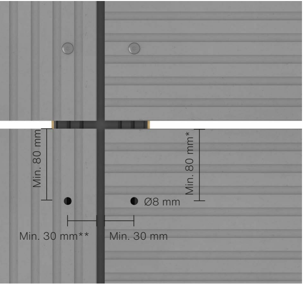
Opmerking! Min. afstand en/of de dichtstbijzijnde rib (bovenste deel van het oppervlak). Fig. 3. Swisspearl Patina Inline randafstanden.
