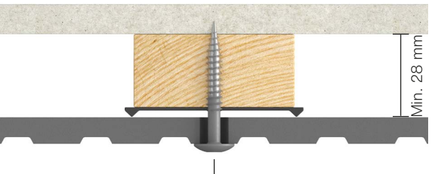
Plaats de schroef in het midden van de bovenkant van de rib. Fig. 2. Swisspearl Patina Inline plaatsing op tussenstijlen.
