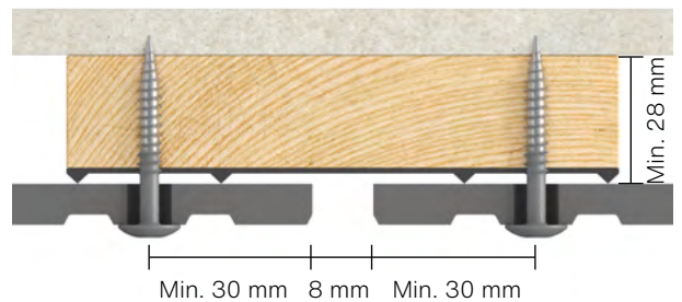
Fig. 1. Swisspearl Patina Inline plaatsing op draaglatten ter hoogte van een voeg.
