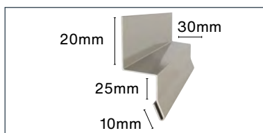
8. Alu waterslagprofiel
