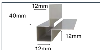
1. Alu buitenhoekprofiel
