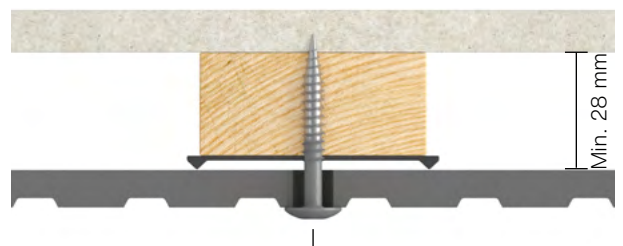
Fig. 2. Swisspearl Patina Inline plaatsing op tussenstijlen.
