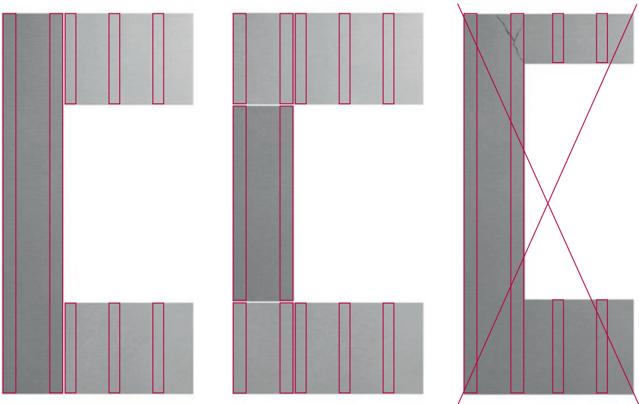
Swisspearl-julkisivulevyjen oikea asennus ikkunoiden, ovien ja aukkojen kohdalla.
