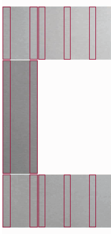
Swisspearl-julkisivulevyjen oikea asennus ikkunoiden, ovien ja aukkojen kohdalla.
