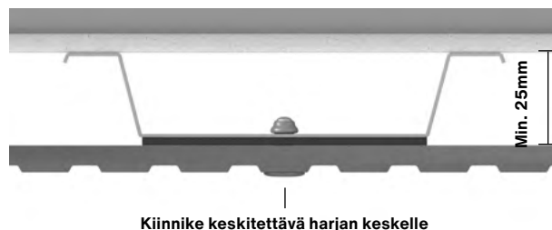
Kuva 2. Swisspearl Patina Inline -levyn asennus profiiliin keskelle
