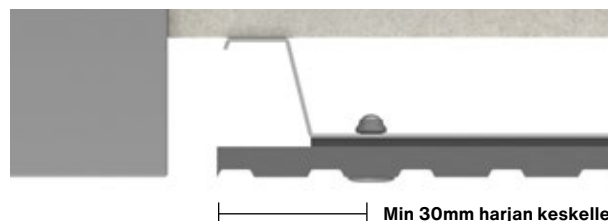
Kuva 4. Mittaan sahatus Swisspearl Patina Inline -levyn asennus
