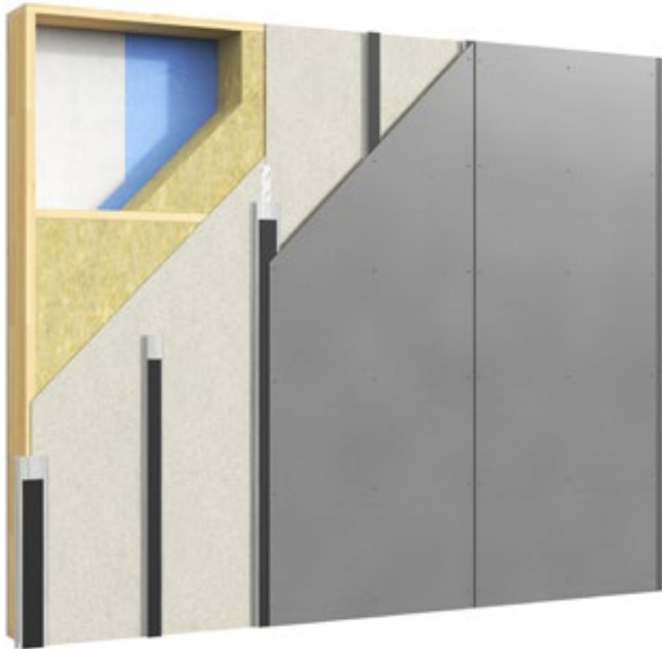
Kevyt seinä pystysuorilla teräsprofiileilla
