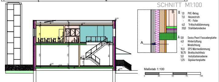
Schnitt M1:100
