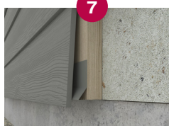
7. Start/ventilationsprofil
