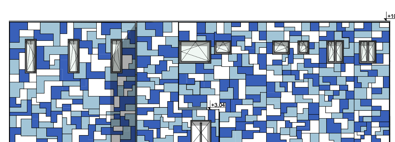
Ansicht Süd M 1:200
