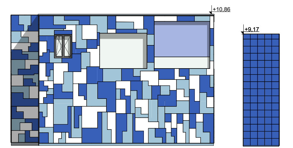
Ansicht Ost M 1:200
