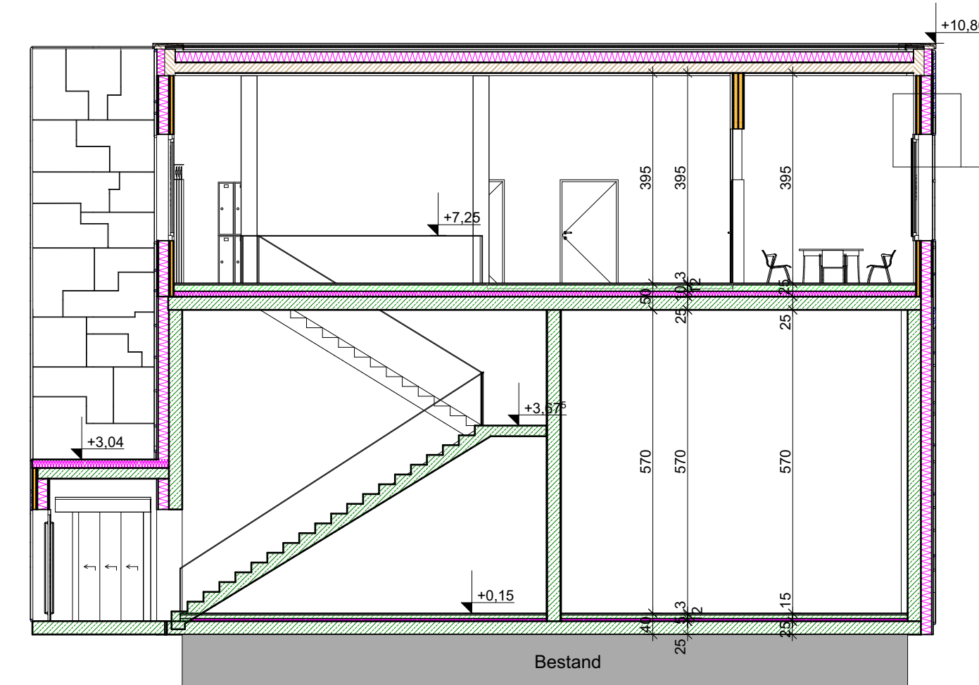
Schnitt M 1:200
