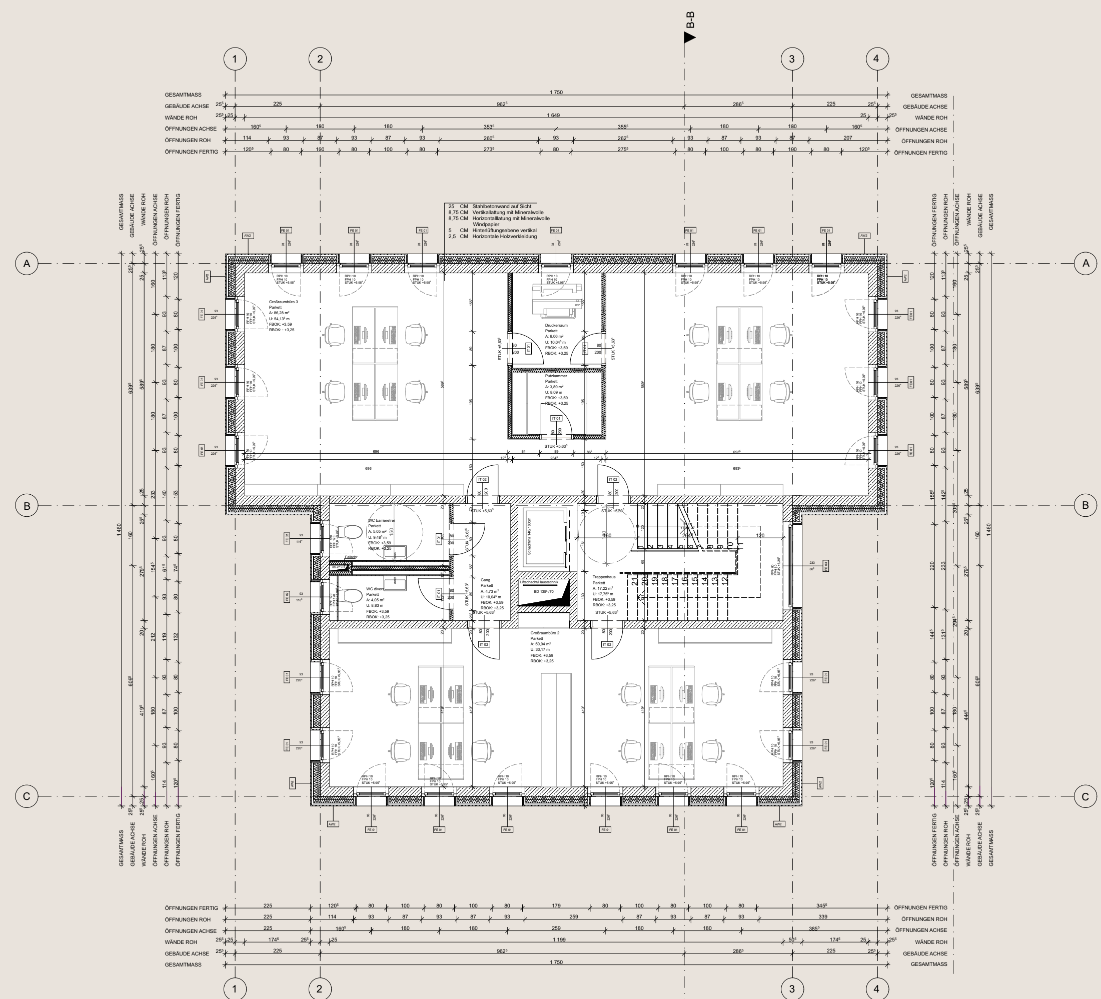
Regelgeschoss M 1:100
