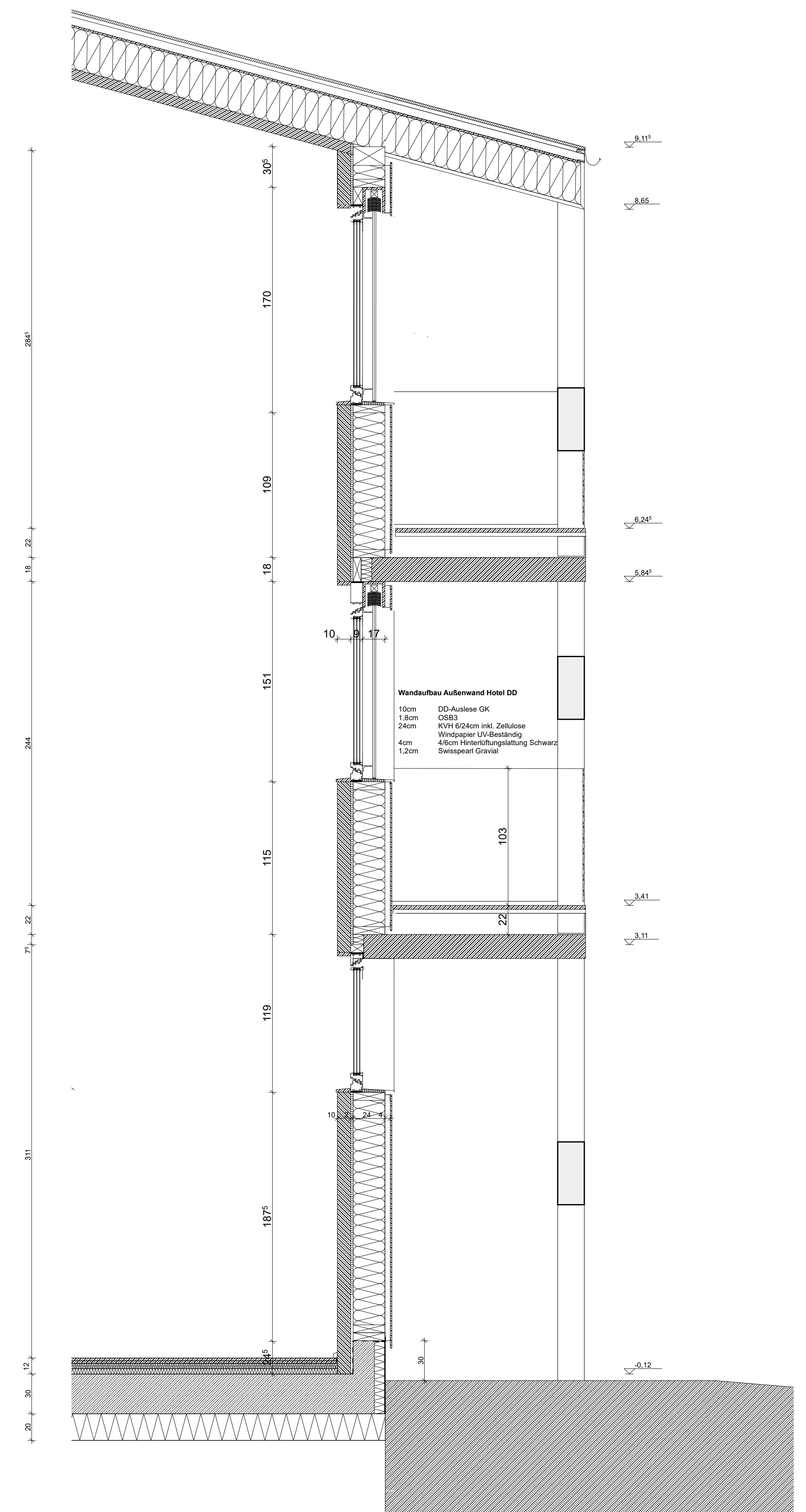
Fassadenschnitt
