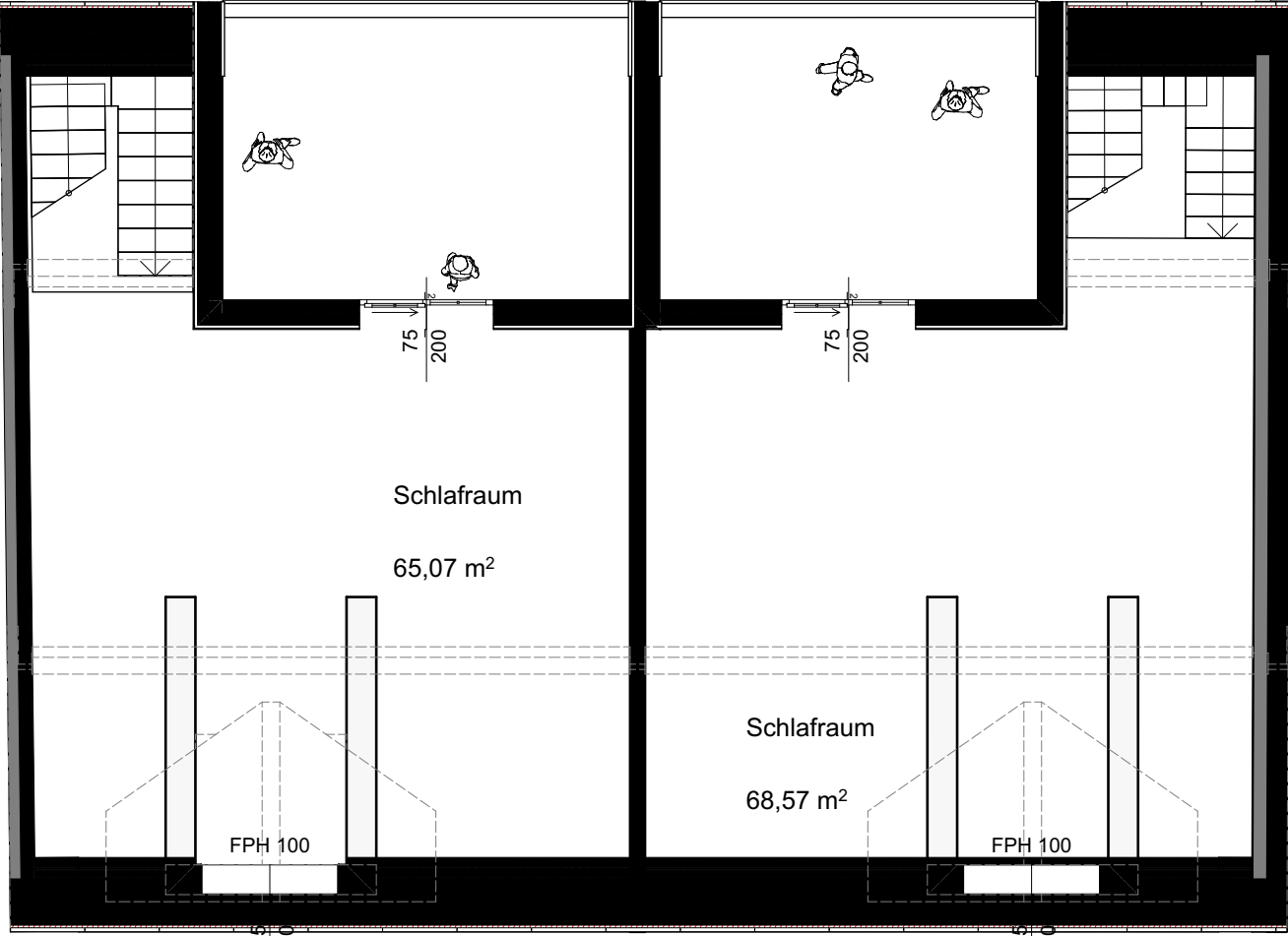
Dachgeschoss 1:100
