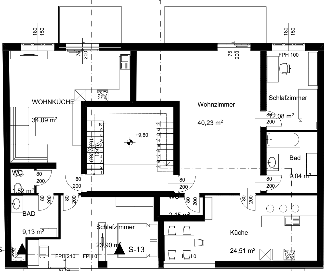
Regelgeschoss 1:100
