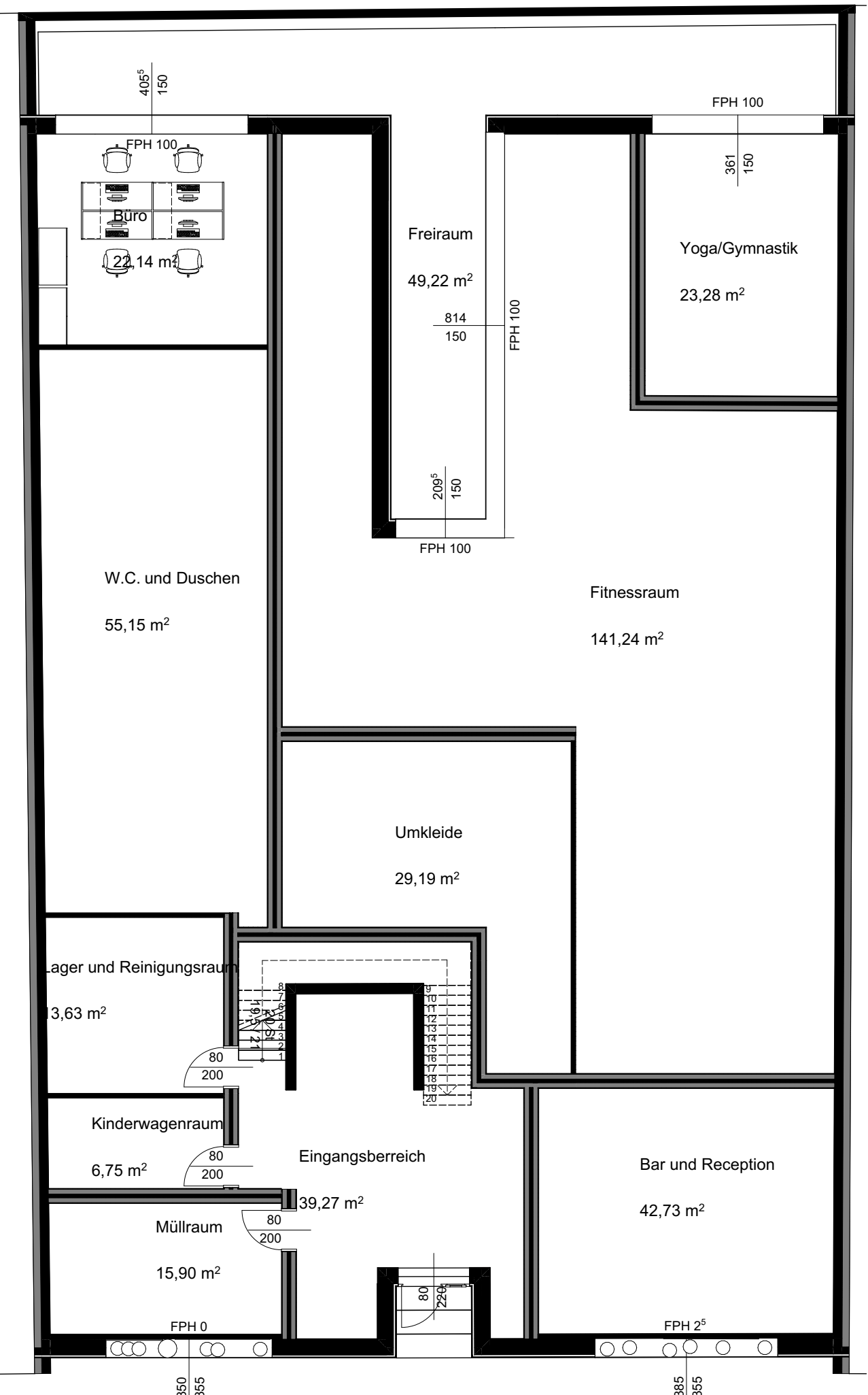
Erdgeschoss 1:100
