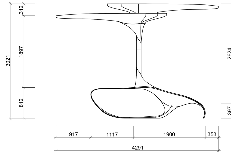
KREUZRISS
