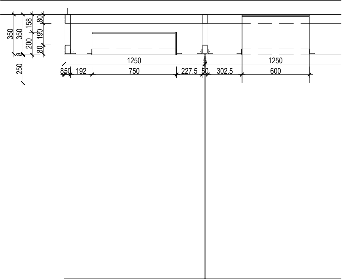
Grundriss Schnitt
