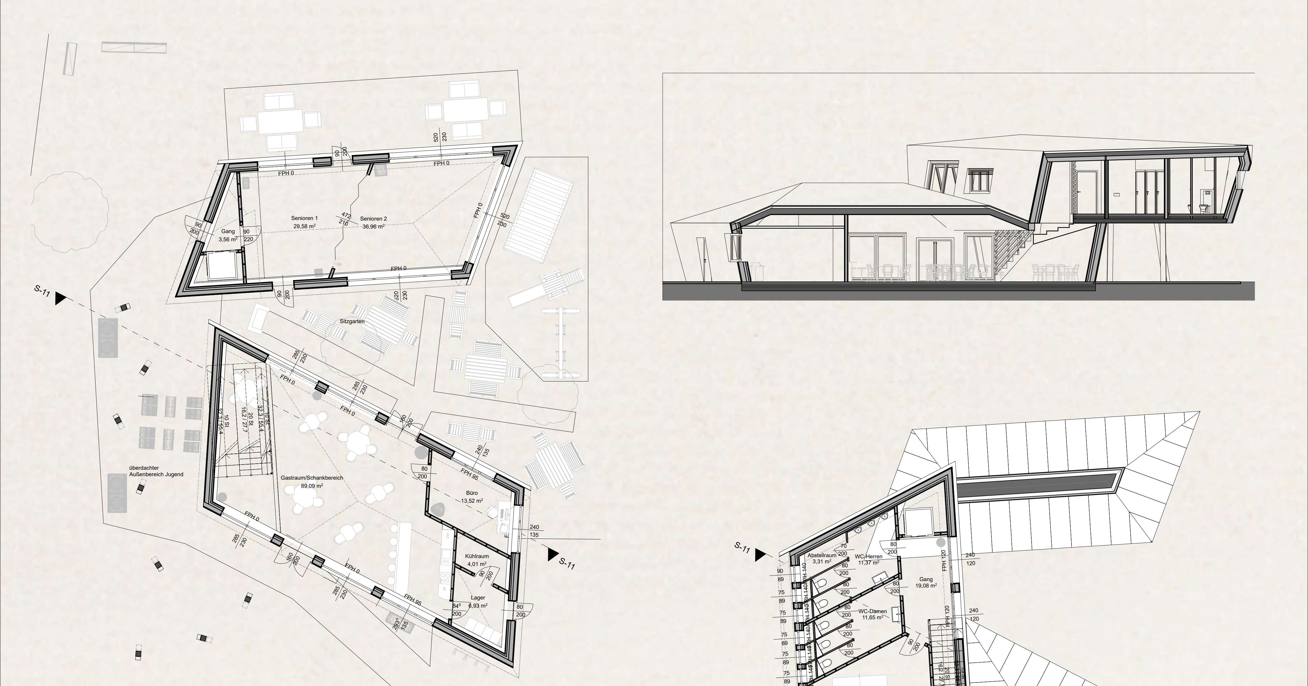
Grundriss EG
