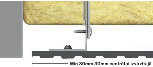
4. attēls Swisspearl Patina Inline uzstādīšana un pēc izmēra sagrieztas plāksnes.
