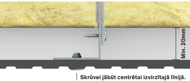
2 attēls. Swisspearl Patina Inline uzstādīšana uz L profila
