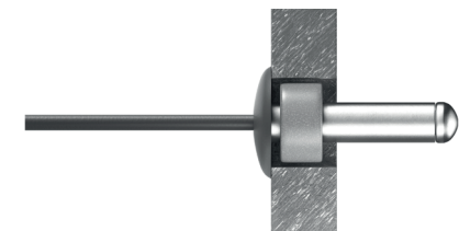
X: Stiprinājuma punkta urbuma diametrs Ø 9 mm. Pie kniedes nostiprināšanas fiksētajā stiprinājuma punktā, tiek izmantots Swisspearl ieliktnis kniežu fiksēto stiprinājumu punktu realizācijai. Pērējie stiprinājumi - slīdošie stiprinājumi.
