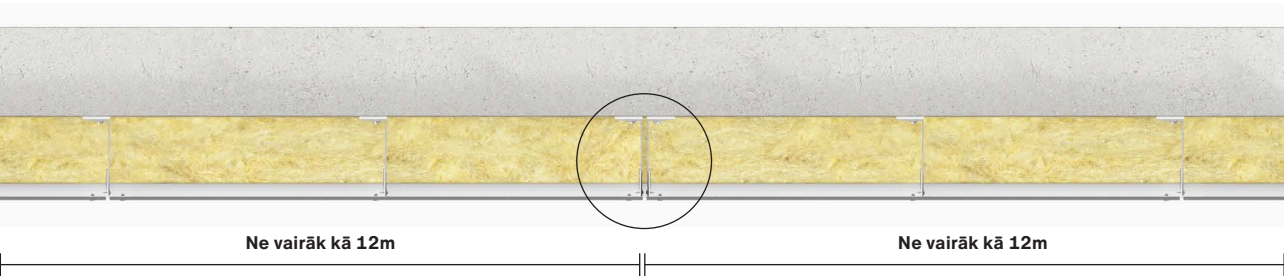
Apakškonstrukcijas taisnums
