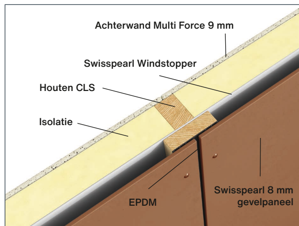
Geventileerde gevel met Windstopper en Swisspearl gevelpanelen
