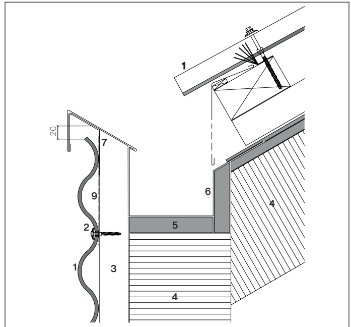
Verlegung horizontal
