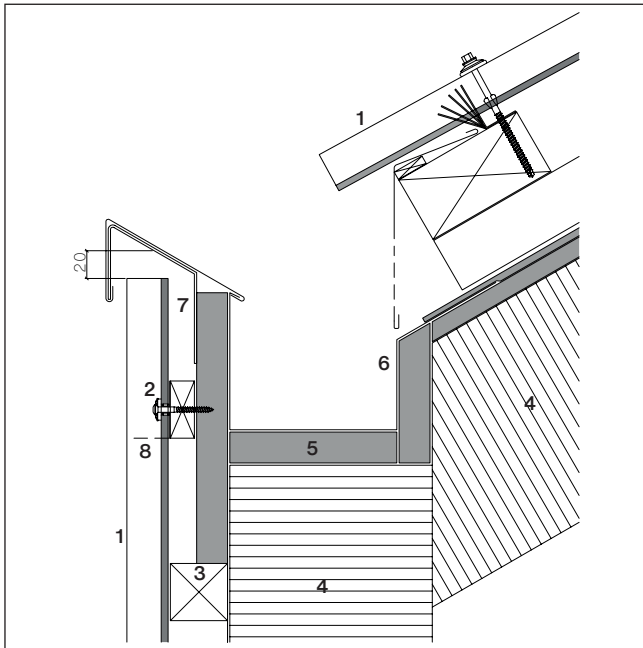
Verlegung vertikal
