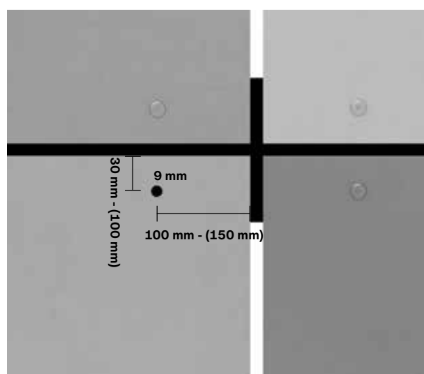
Fig. 4 Horisontal støtte
