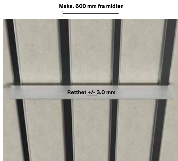
Fig. 1 Underkonstruksjonens retthet
