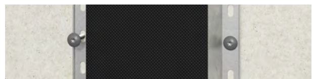
Fig. 3 I skyvepunktene monteres Swisspearl monteringsprofiler med to skruer mot hverandre for å unngå deformasjon i stålet.
