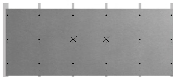
Fig. 3 Eksempel: Horisontalt monterte plater med fi re mellomliggende stålfiler.
