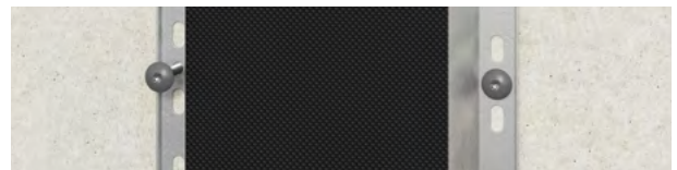
Fig. 2 Swisspearl monteringsprofiler monteres i festepunktene med to skruer mot hverandre for å unngå deformasjon i stålet.
