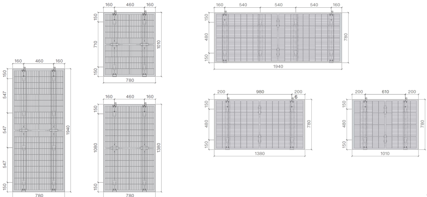
Vertikale Anordnung
