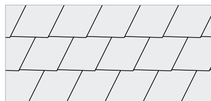
Einfachdeckung Rhombus 400 × 440 mm
