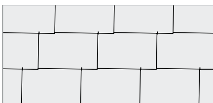
Einfachdeckung Rechteck 600 × 400 mm
