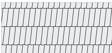
Einfachdeckung Steinschindel 194 × 385 mm
