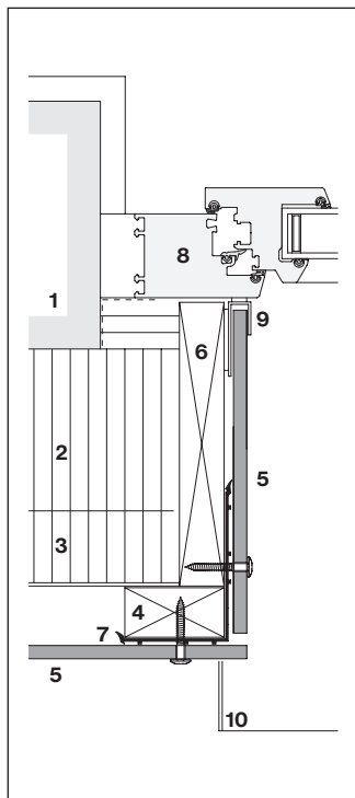
Vertikaalne ristlõige
