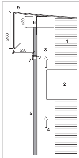
Räästaplekid
