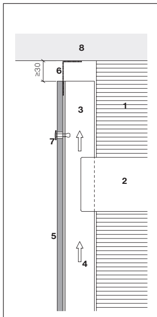
Ühendus ripplae/horisontaaltarindiga
