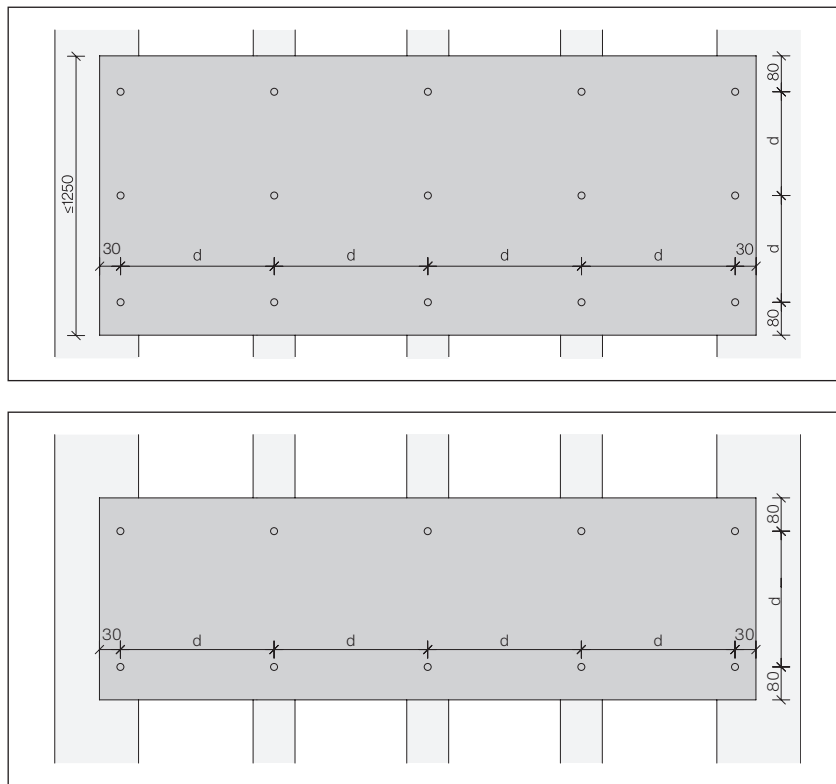
Swisspearl Largo horisontaalpaigaldus
