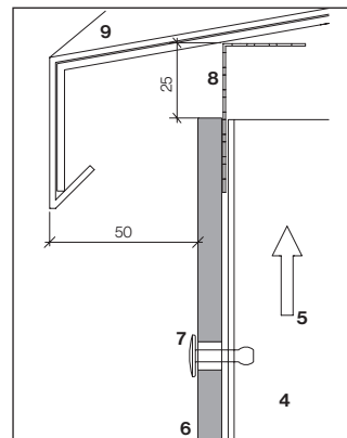
Akna veepleki detailjoonis
