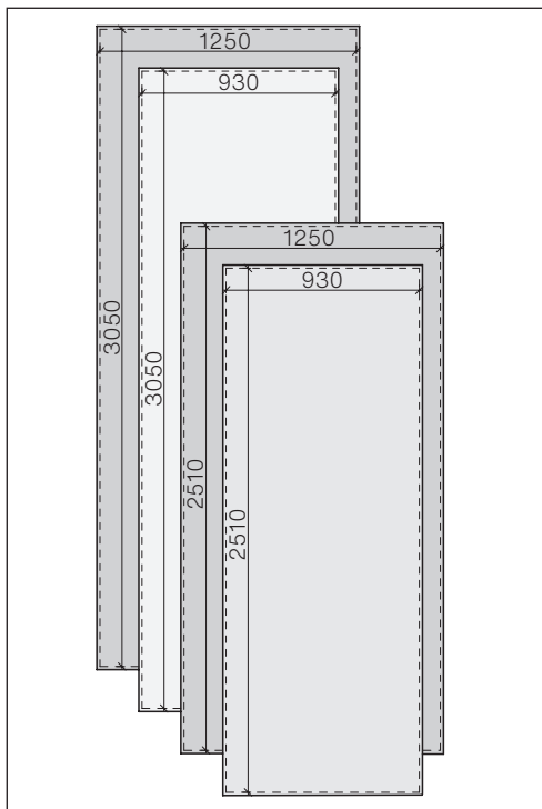
8 mm ja 12 mm paksused plaadid – maksimaalsed plaadimõõdud
