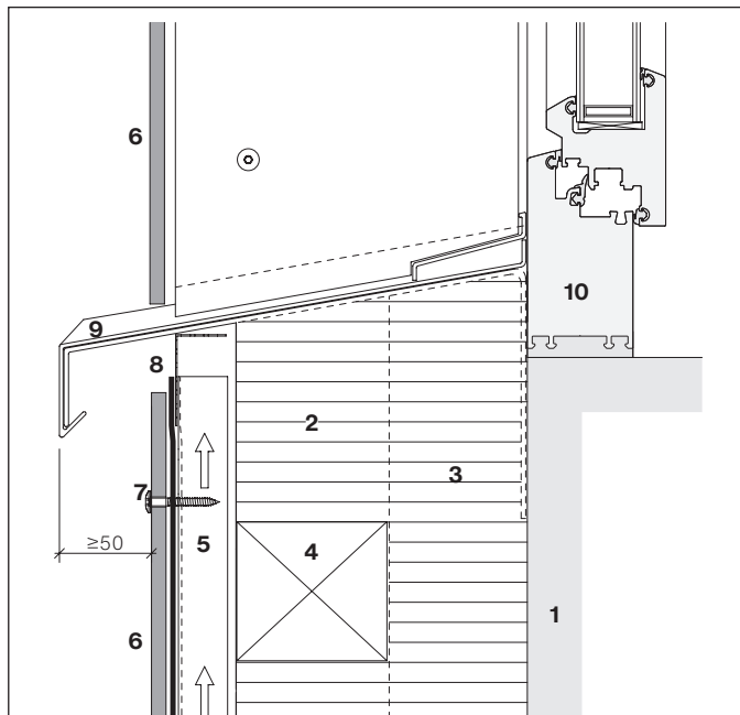
Akna veeplekk
