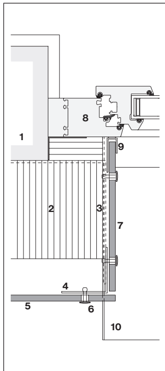
Horisontaalne ristlõige
