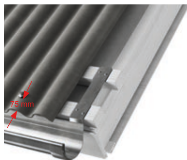
Joonis 2. Katuseräästa juures on kaugus plaadi servast kuni esimese kinnituspunkti vähemalt 75 mm.
