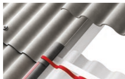
Joonis 31. Laineplaatide kõrvale paigaldatud läbipaistvad plaadid Eurolux; piki- ja ristsuunaline ülekate.
