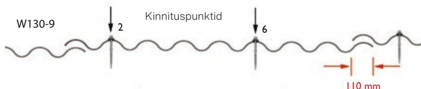
Joonis 24a. Plaatide W130-9 kinnituspunktid on 2. ja 6. laine harjal. Siin on kujutatud katuseviilu katmist vasakult paremale.
