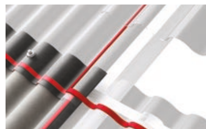
Joonis 32. Kõrvutiasetsevate läbipaistvate plaatide Eurolux ühendamine; piki- ja ristsuunaline ülekate.
