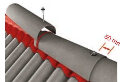
Joonis 35. Poolsilindri kujulise harjadetaili paigaldamine.
