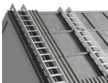
Joonis 17. Näide redelite riputamisest laineplaatidest katusekatte paigaldamisel.
