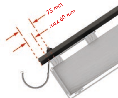
Joonis 20. Kaugus kinnituspunktist plaadi alumise servani on 75 mm.
