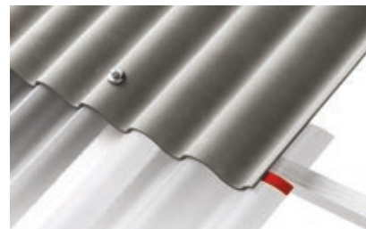
Joonis 28. Laineplaatide EuroFala alla paigaldatud läbipaistvad plaadid Eurolux; ristsuunaline ülekate.
