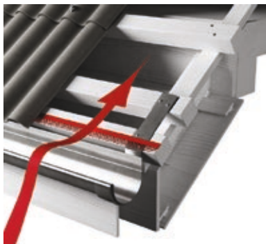
Joonis 5. Katuseräästas: tuulutusavade pindala 1 jooksva meetri kohta: plaadid W130-9 – 120 cm 2 .
