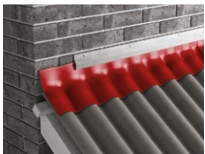
Joonis 44. Katuseviilu ja hoone seina ühenduskoha ehitamine.
