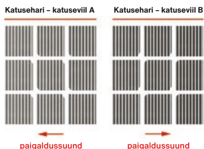
Joonis 13. Plaatide nurkade lõikamine vastavalt nende paigaldussuunale.
