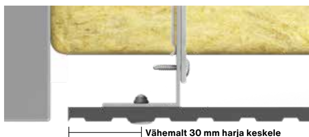
Pilt 4. Mõõtusaetud Swisspearl Patina Inline plaadi paigaldamine
