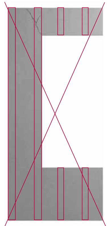
Swisspearli fassaadiplaatide vale paigaldus akende, uste ja avade juures.
