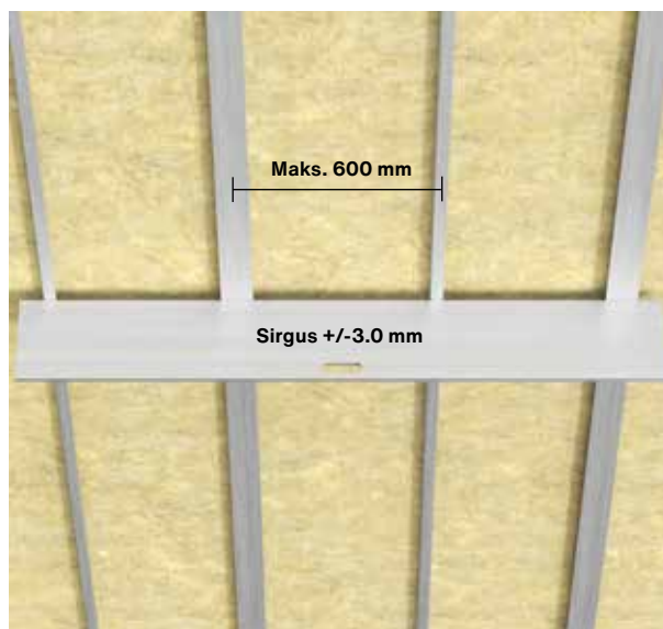
Aluskonstruksiooni sirgus
