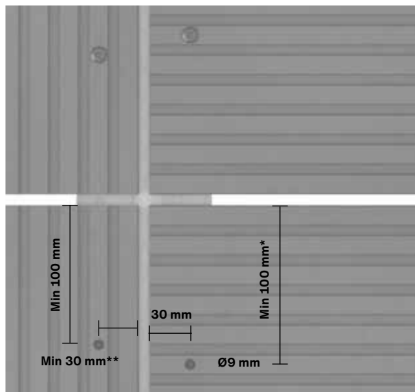
Pilt 3. Swisspearl Patina Inline servakaugused NB! Minimaalne kaugus ja/või järgmine hari.
