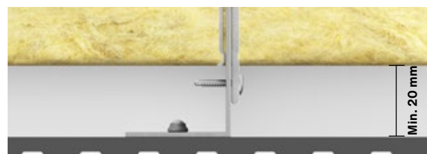
Pilt 2. Swisspearl Patina Inline plaadi paigaldamine L-profiilile
