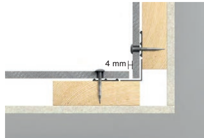
Sisänurkkaratkaisu avoimella liitoksella
