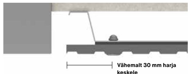
Pilt 4. Mõõdusaetud Swisspearl Patina Inline plaadi paigaldamine
