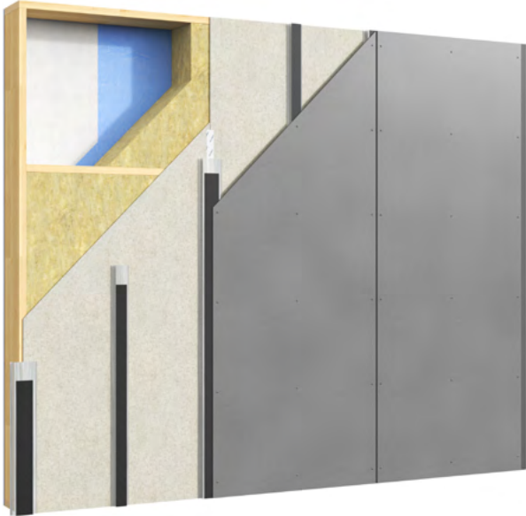
Kergsein terasest püstprofiilidega
