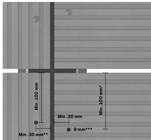
Pilt 3. Swisspearl Patina Inline plaadi paigaldamisel kasutatavad servakaugused
