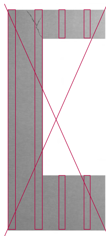
Swisspearli fassaadiplaatide vale paigaldus akende, uste ja avade ümber.
