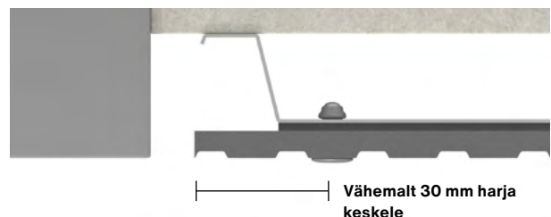
Pilt 4. Mõõtsaetud Swisspearl Patina Inline plaadi paigaldamine
