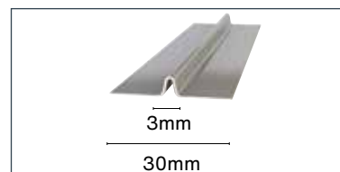
7. Alu voegprofiel
