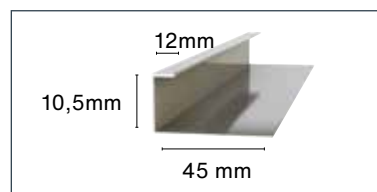
10. Alu eindprofiel
