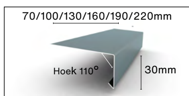
6. Alu raamdorpelprofiel
