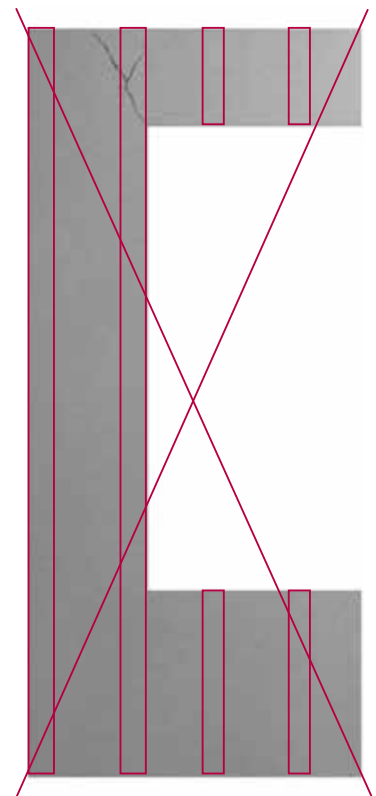
Nepareiza Swisspearl fasādes plākšņu montāža pie logiem, durvīm un ailēm.
