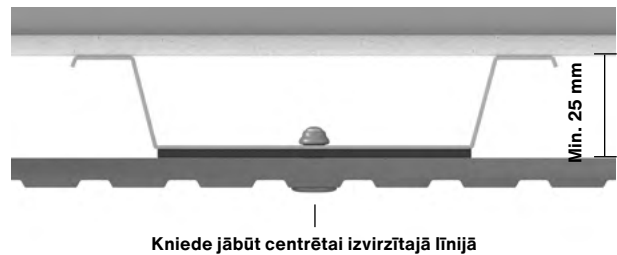
2. attēls Swisspearl Patina Inline - stiprināšana uz starposma balsta
