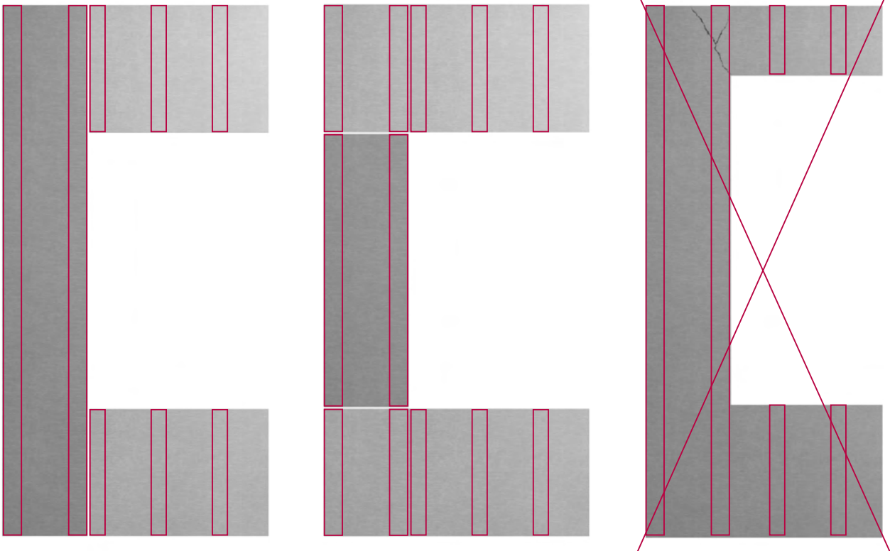
Pareiza Swisspearl fasādes plākšņu montāža pie logiem, durvīm un ailēm.
