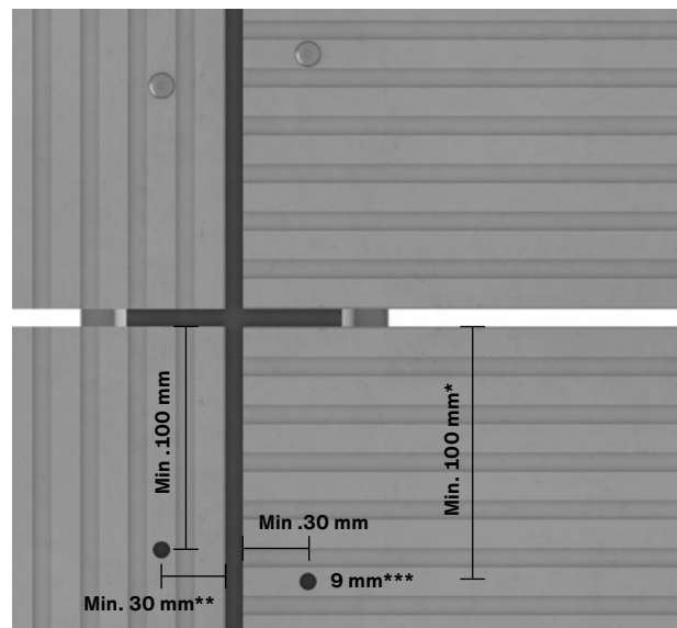
3. attēls Swisspearl Patina Inline Malu attālumi Piezīme! Minimālais attālums un/vai tuvākā izvirzītā ***9 mm urbums kniedēm
