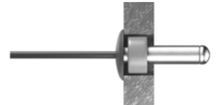
X : Stiprinājuma punkta urbuma diametrs Ø 9 mm. Pie kniedes nostiprināšanas fiksētajā stiprinājuma punktā, tiek izmantots Swisspearl ieliktnis kniežu fiksēto stiprinājumu punktu realizācijai.
