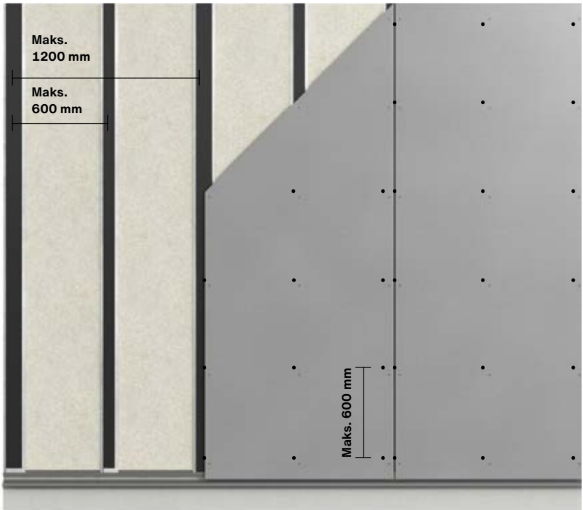
Swisspearl Patina fasādes plāksnes ustādītas uz vertikālas tērauda apakškonstrukcijas
