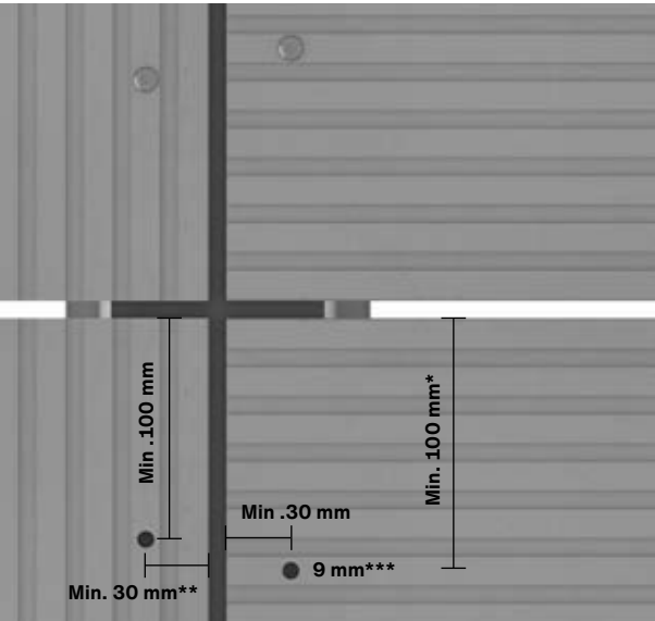
3. attēls Swisspearl Patina Inline Malu attālumi Piezīme! Minimālais attālums un/vai tuvākā izvirzītā ***9 mm urbums kniedēm
