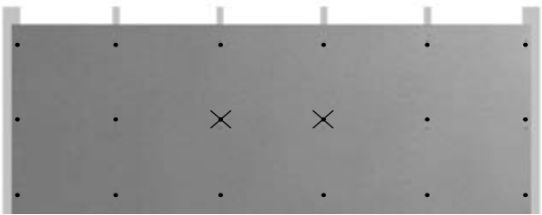
Piemērs: horizontāli piestiprinātas plāksnes ar četriem profiliem plāksnes vidusdaļā.
