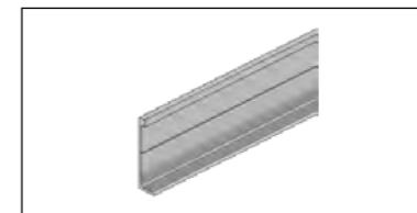
Swisspearl Plank Connect -aloitusprofiili, pystyasennus Suulakepuristettu alumiini Paksuus 1,1 mm Pituus 3 000 mm
