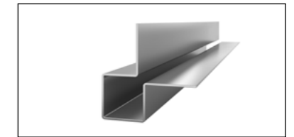
Swisspearl ulkokulmaprofiili, pieni Maalattu, alumiini Paksuus 1,0 mm Pituus 3 000 mm
