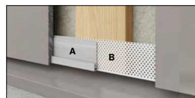
Kuva 7 A. Swisspearl Plank Connect -aloitusprofiili B. Swisspearl tuuletusprofiili
