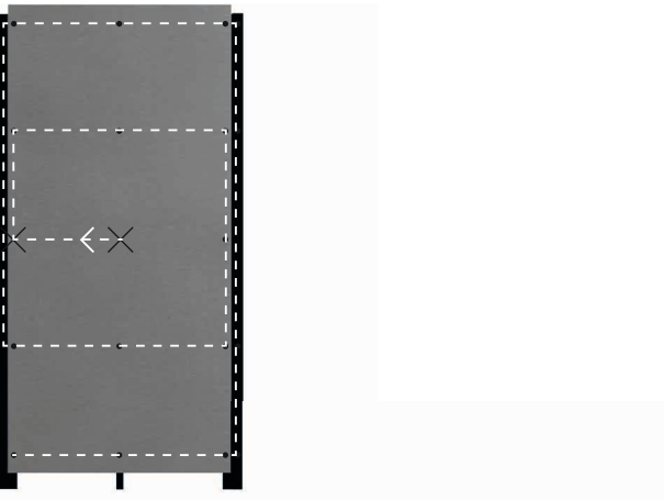
Illustrasjon av korrekt montering med fast punkt (X).
