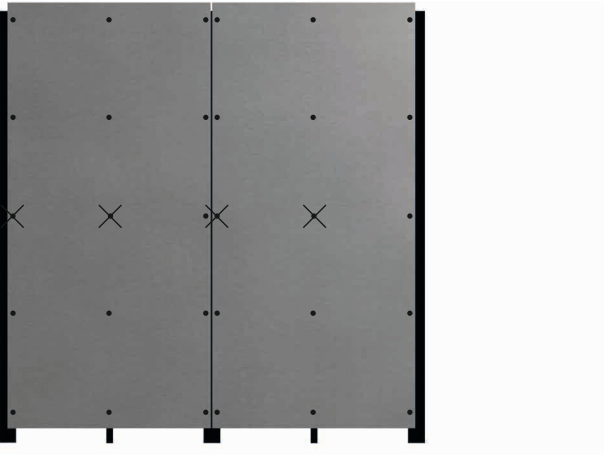
Eksempel: Stående montering med fast punkter (X).
