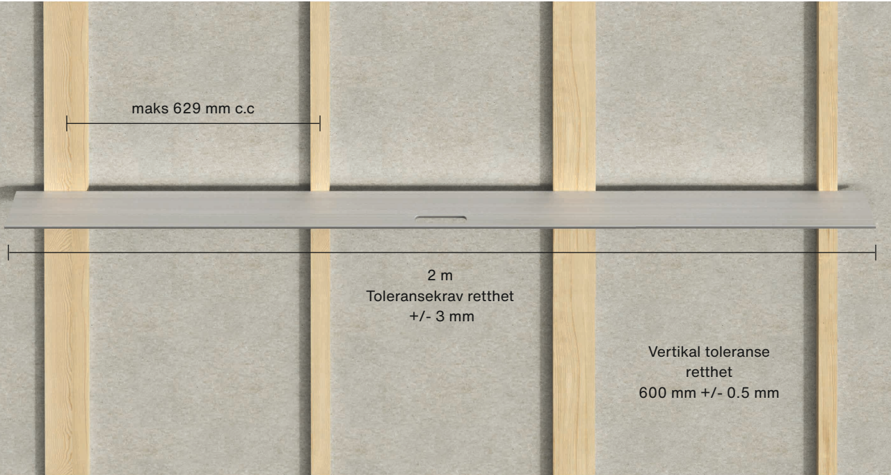
Retthet av underkonstruksjon
