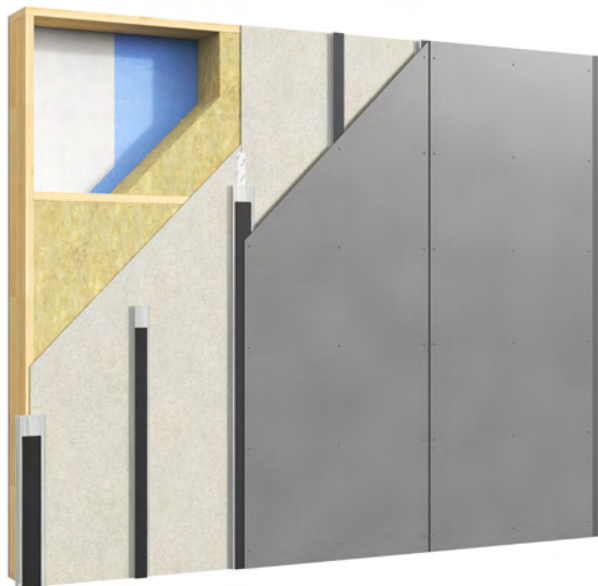
Karkasinė siena su vertikaliai išdėstytais plieniniais profiliais
