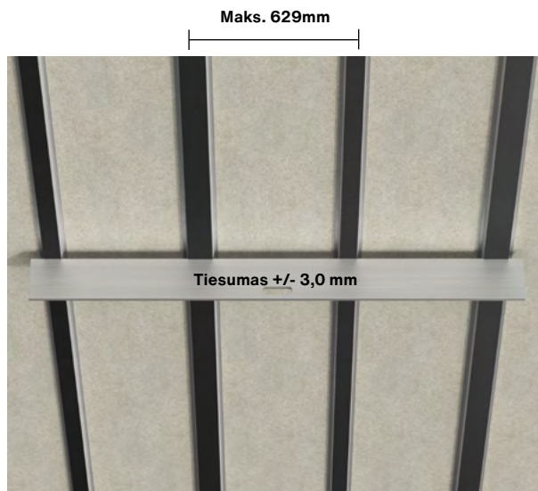
Pagrindo konstrukcijos tiesumas
