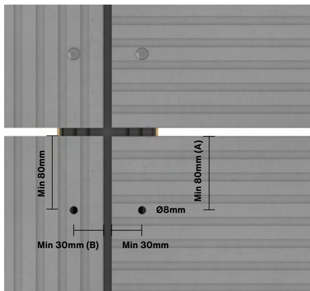
Pilt 3. Swisspearl Patina Inline plaadi servakaugused. NB! Minimaalne vahemaa ja/või sellest järgmine hari.
