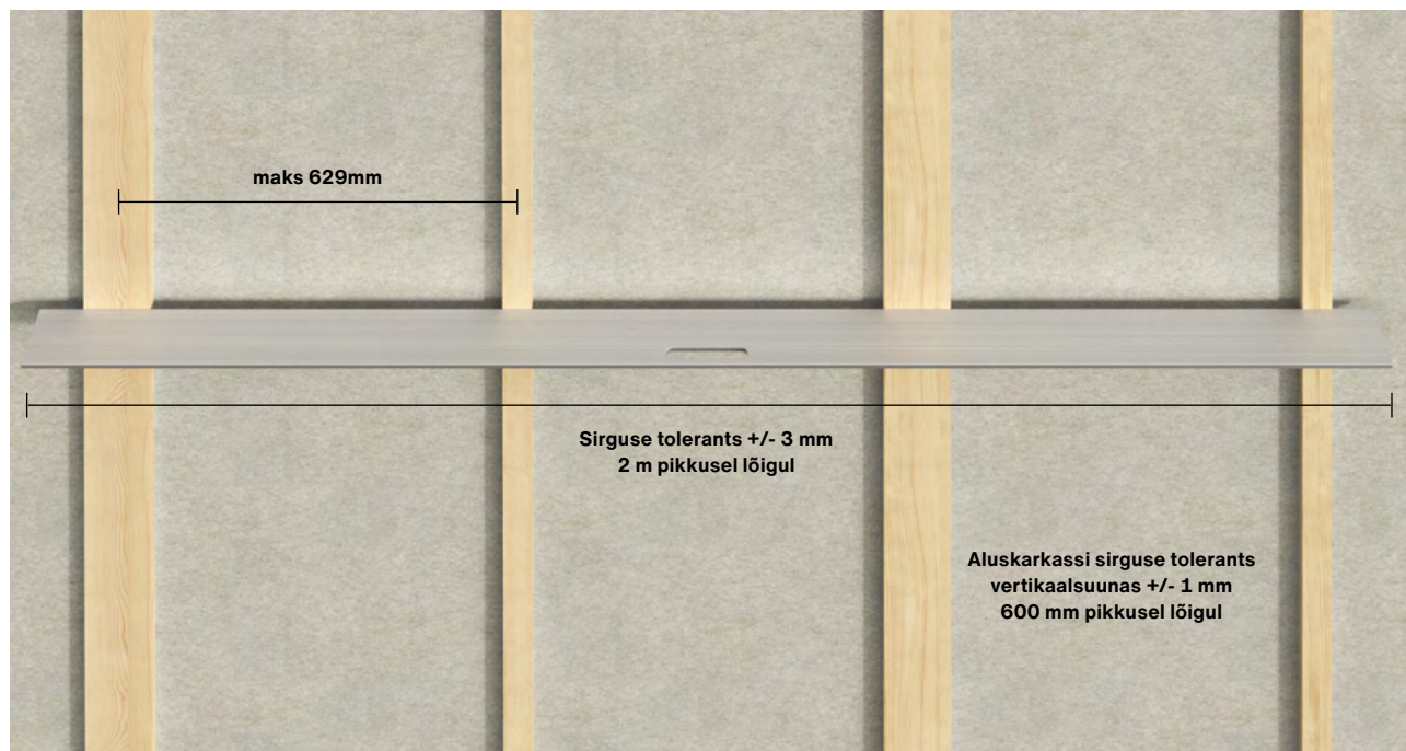
Aluskarkassi loodimine
