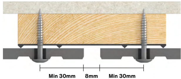
Pilt 1. Swisspearl Patina Inline plaadi paigaldamine püstvuugiga sõlmes.
